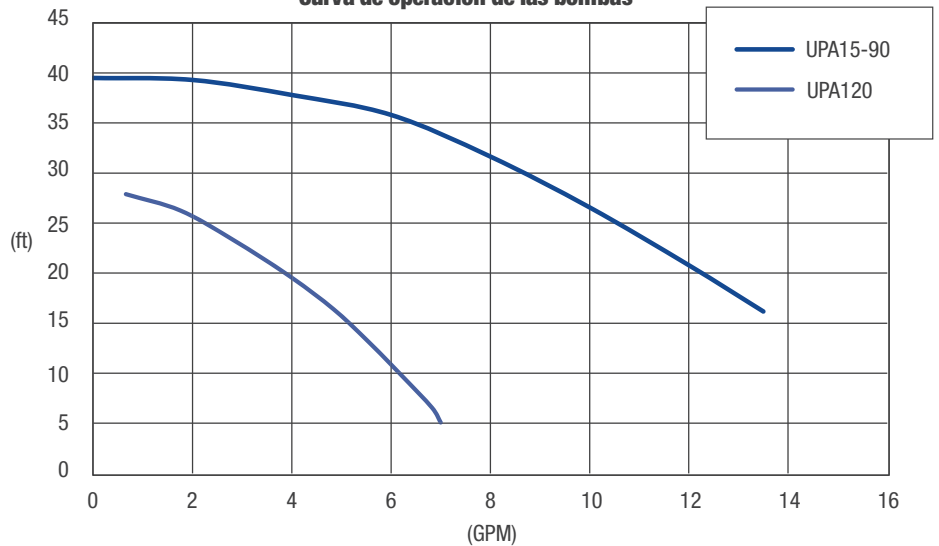
Curva de operación de las bombas
