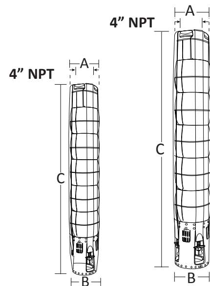
Acoplamiento NEMA 4"
